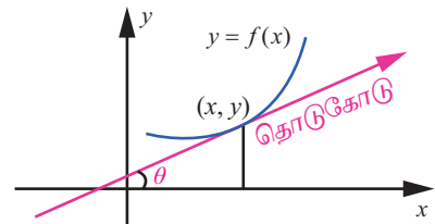
வளைவரையின் சாய்வு \tan(\theta) படம் 7.2
